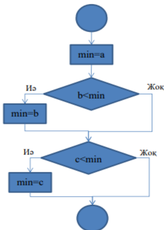
Сурет 38 – Үш санның арасынан ең кіші санды анықтау алгоритмы (үшінші әдіс)
