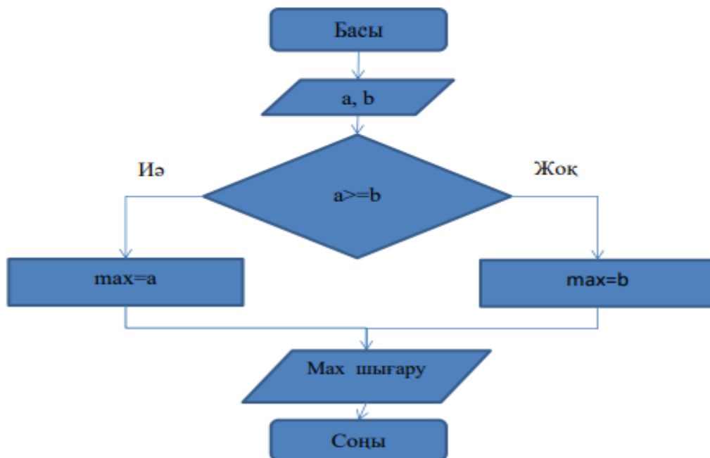
Сурет 35 – Екі санның арасындағы ең үлкен санды табу алгоритмы
