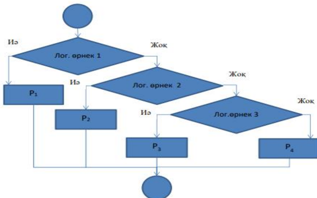
Сурет 34-Көп мағыналы бұтақтардың блок-схемасы
