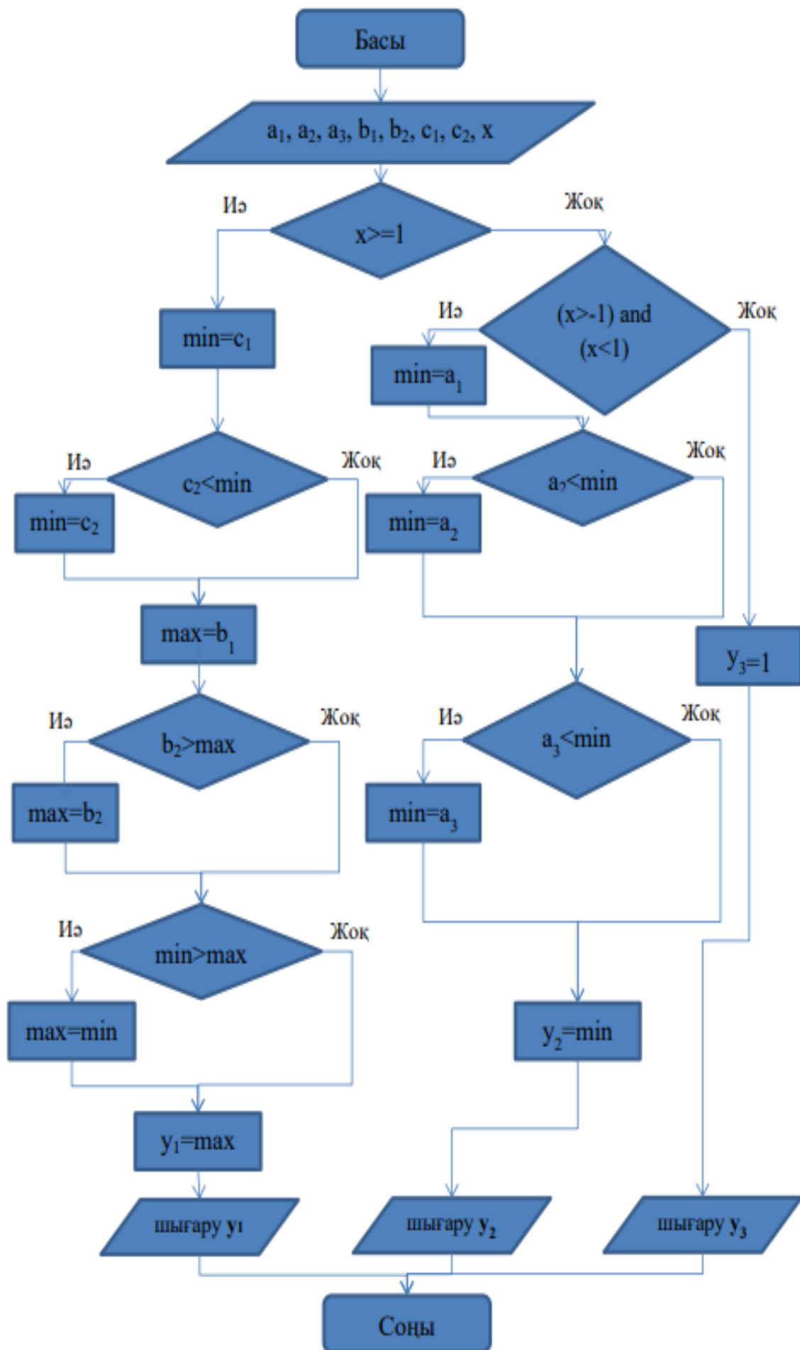
Сурет 39 – 4Алгоритм решения задачи 4.3
