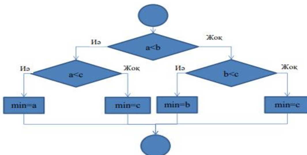
Сурет 36 – Үш санның арасынан ең кіші санды анықтау алгоритмы (бірінші әдіс)
